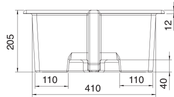
SEZIONE A-A
