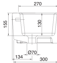
SEZIONE A-A
