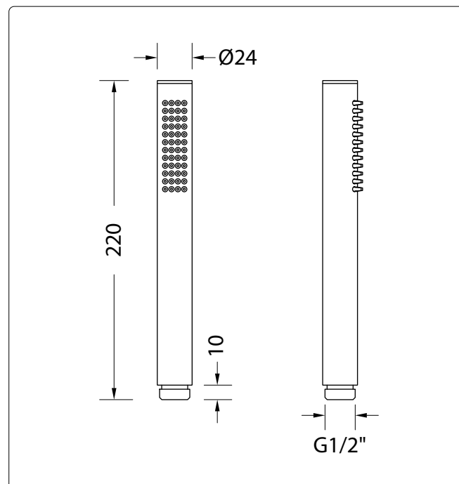
DISEGNO - DRAWING
